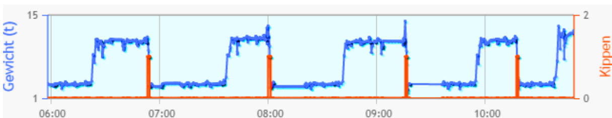
Statistik-Diagramm Korrelation Gewicht und Kippvorgang.
